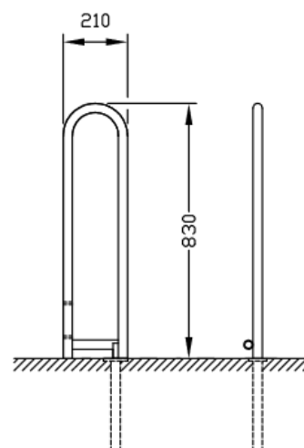
MOD.182-Endelement
