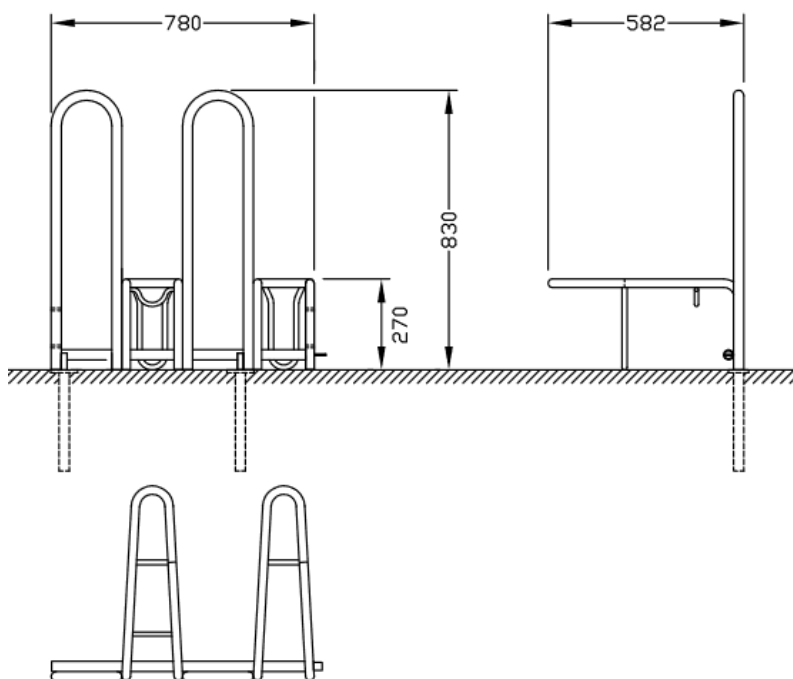
MOD.182-Grundelement
